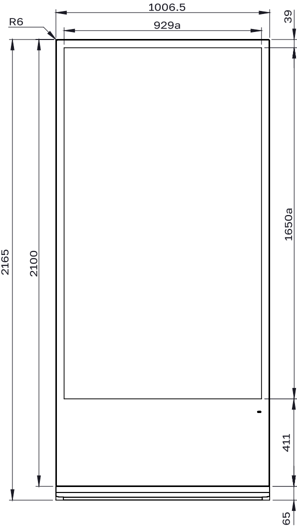
СХЕМА ДИСПЛЕЯ (ВИД СПЕРЕДИ)
