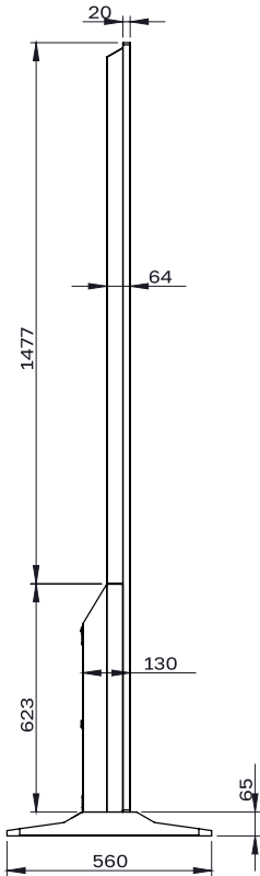
СХЕМА ДИСПЛЕЯ (ВИД СЛЕВА)
